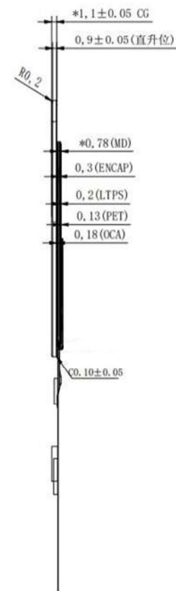
側面図
