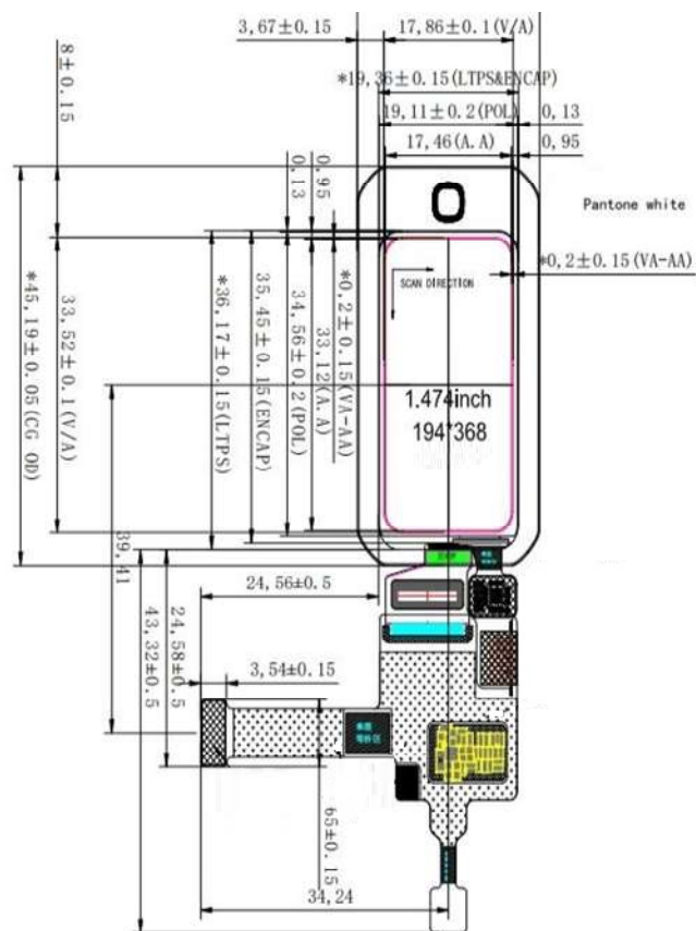
正面図
